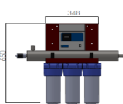
Encombrement du Skid Ecostream 2/4/6
